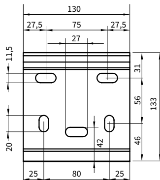
vooraanzicht muursteun
