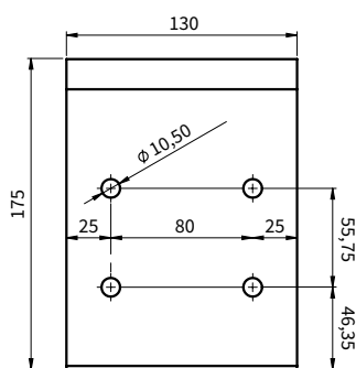
vooraanzicht plafondsteun
